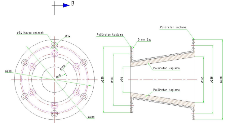
B-B Kesiti
