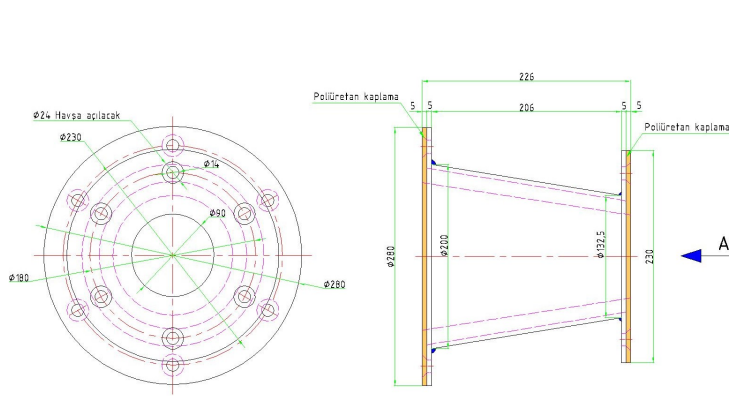
A'dan Görünüş
